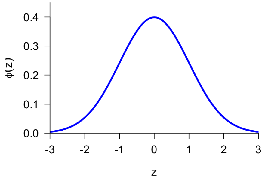
Densidade N(0,1)
