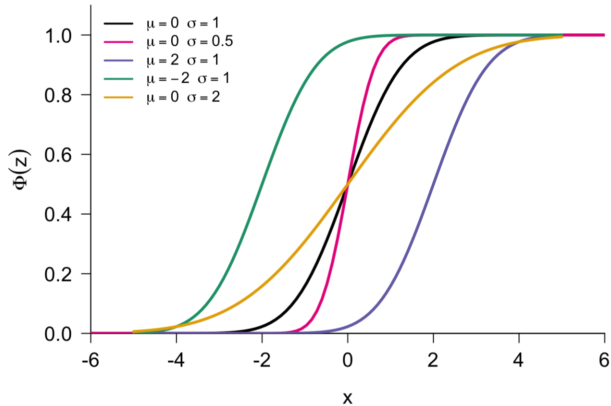
Função de Distribuição Acumulada
